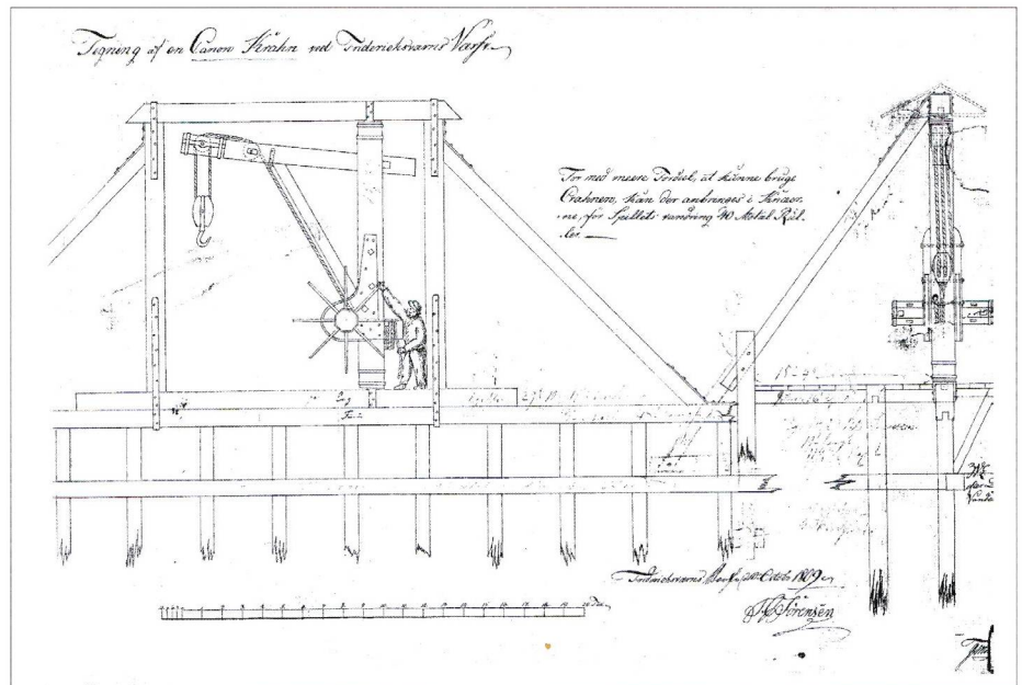
Kran fra 1809.
