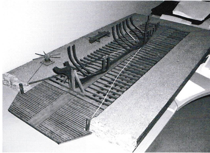
Modell av Fregattbeddingen
